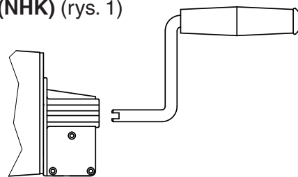
Rys. 1: Awaryjne uruchamianie ręczne NHK Standardowa korba ręczna
